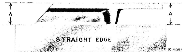
Fig. 23. Perfect Knife Edge
